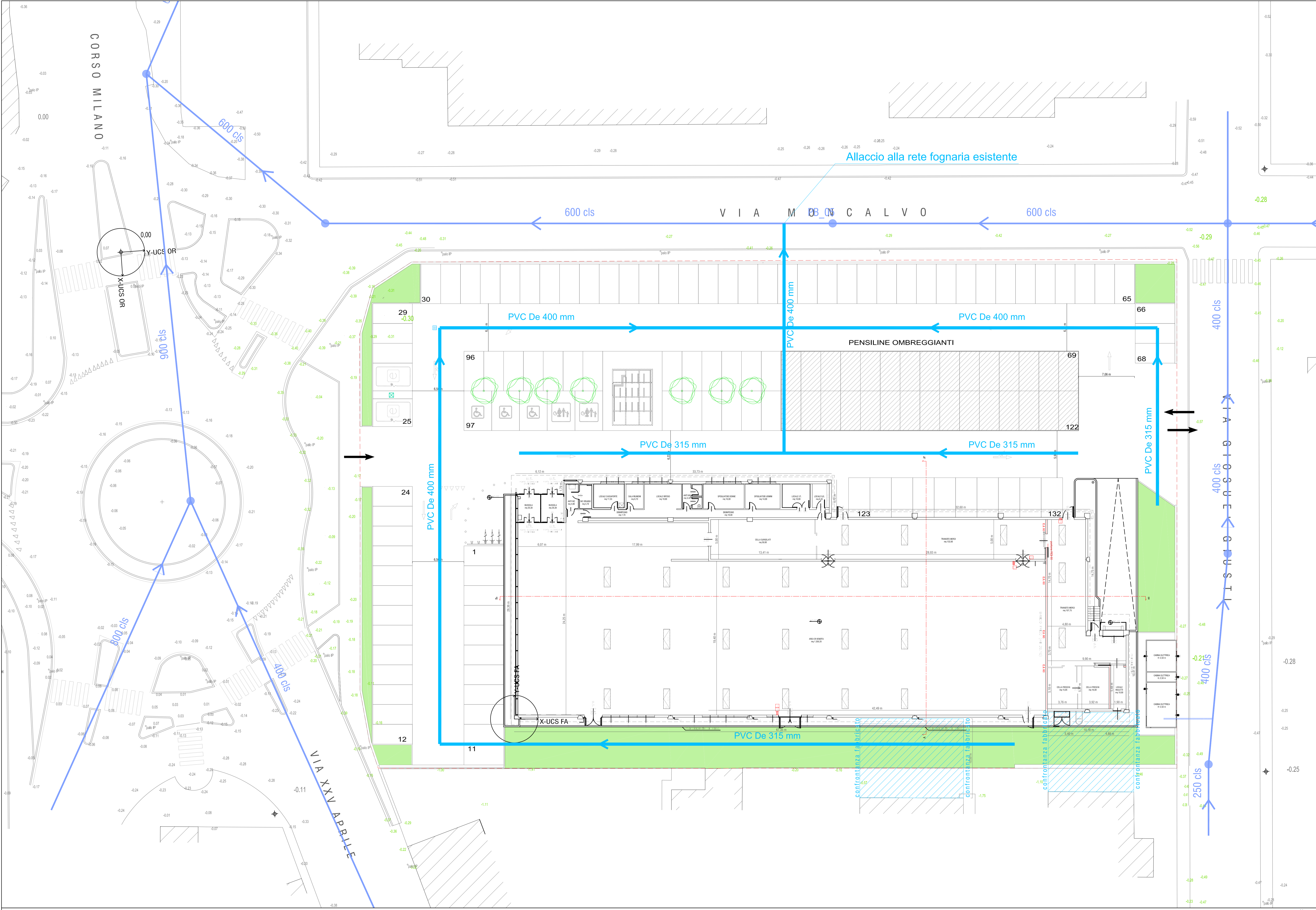
PLANIMETRIA GENERALE
