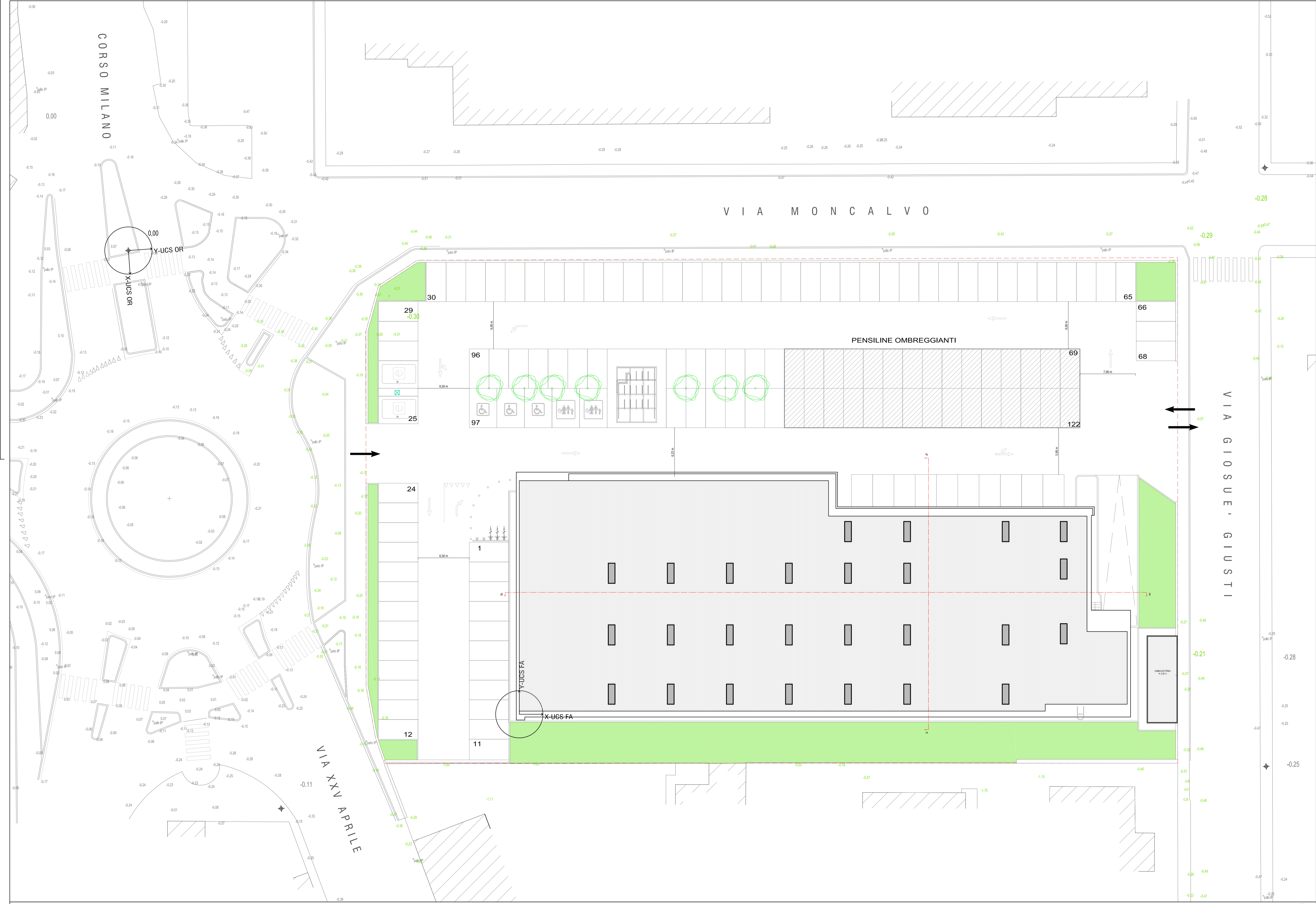
PIANTA DELLE COPERTURE
