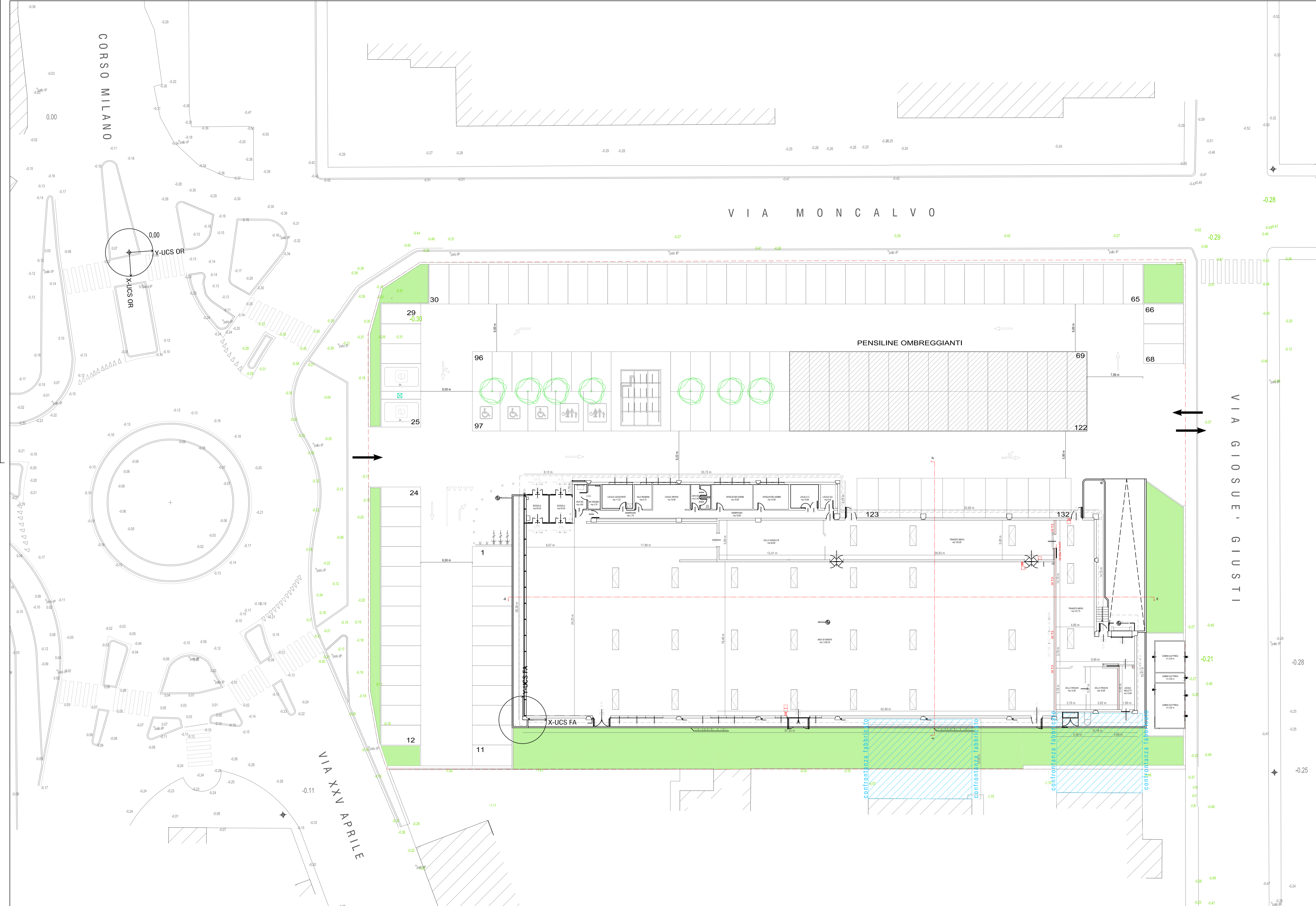
PLANIMETRIA GENERALE
