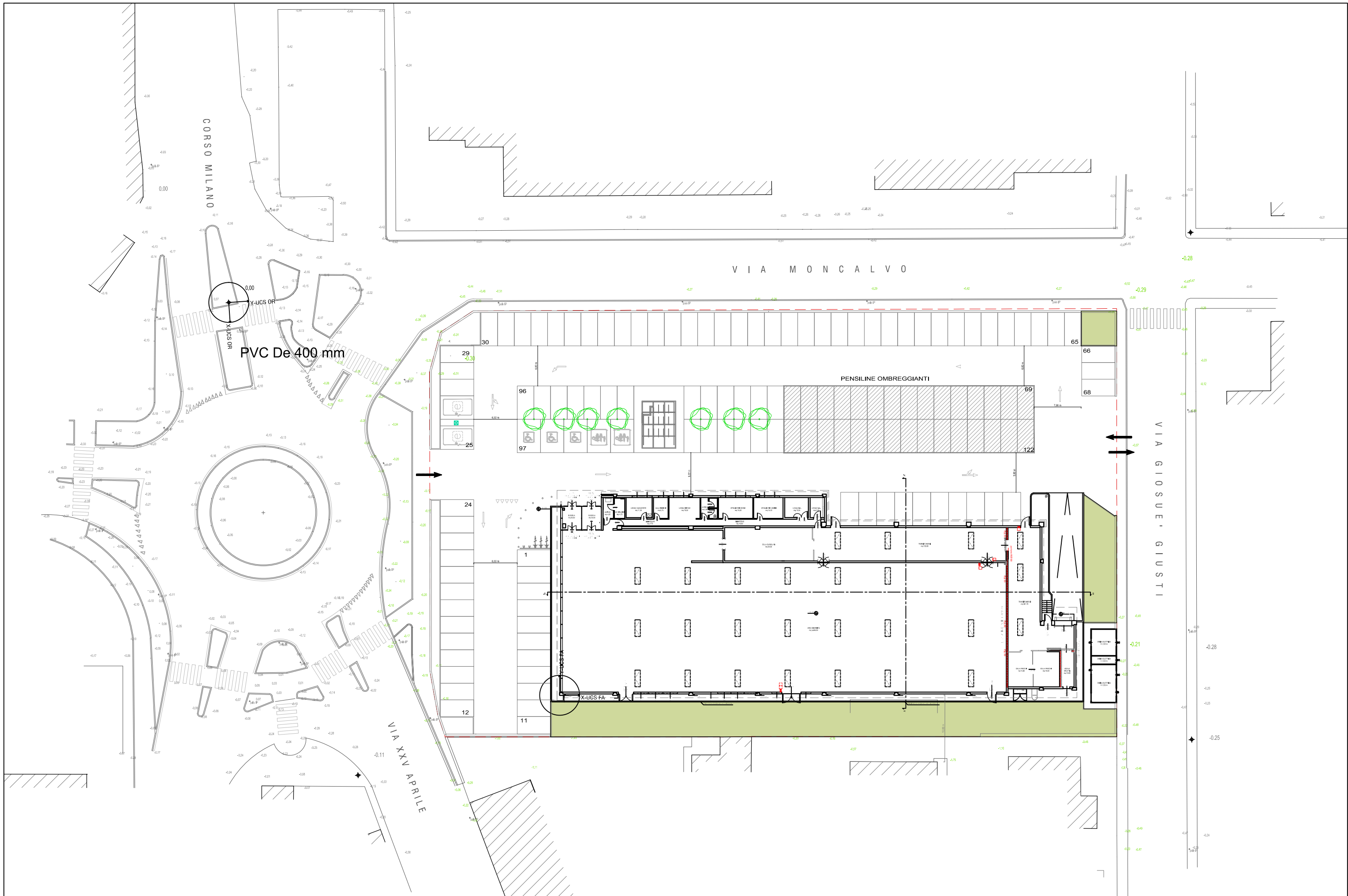
TAVOLA 07 PLANIMETRIA DI PROGETTO
